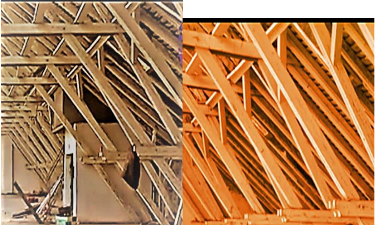
A tetőtér fa szerkezete
